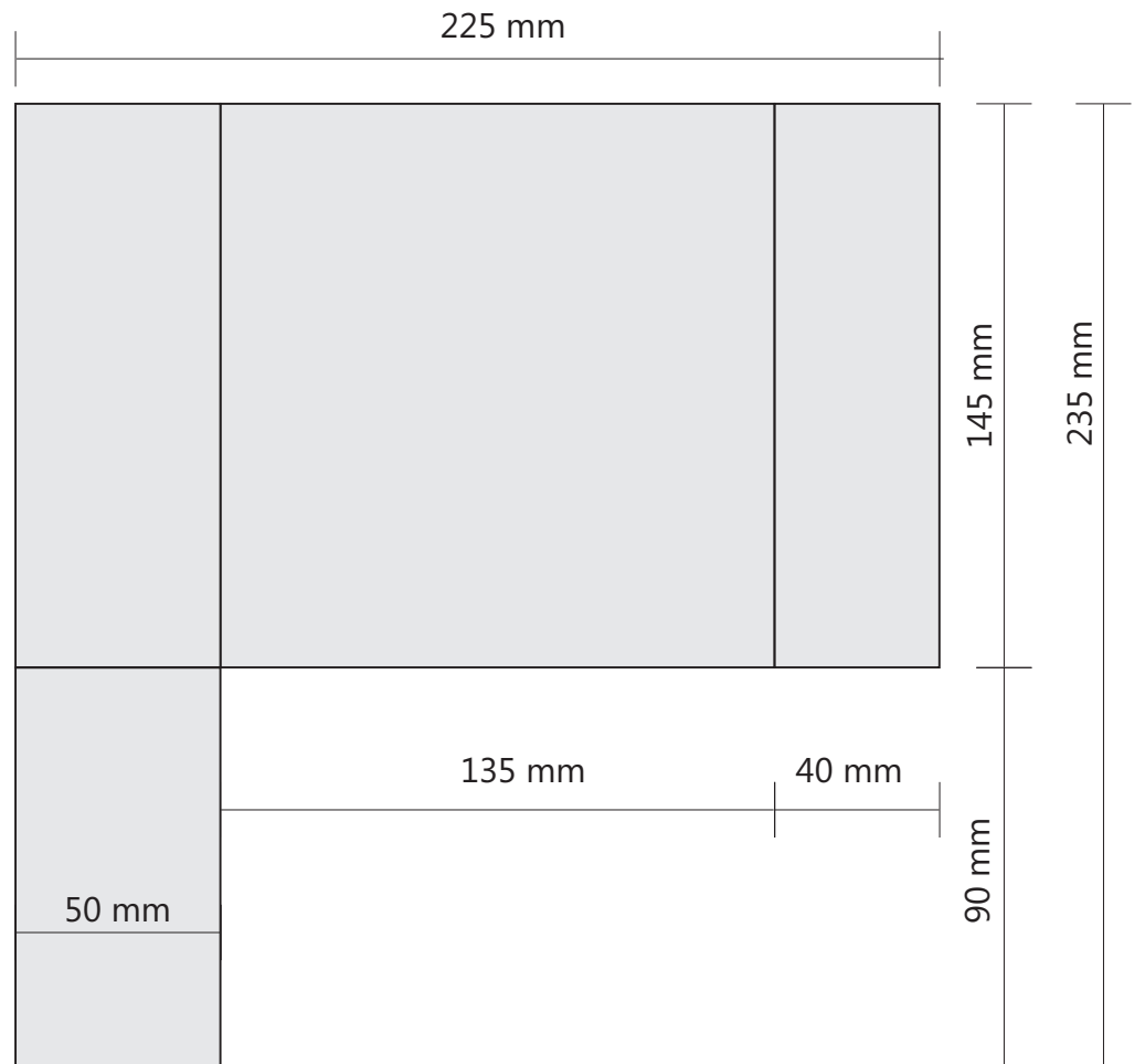
Seitenansicht
