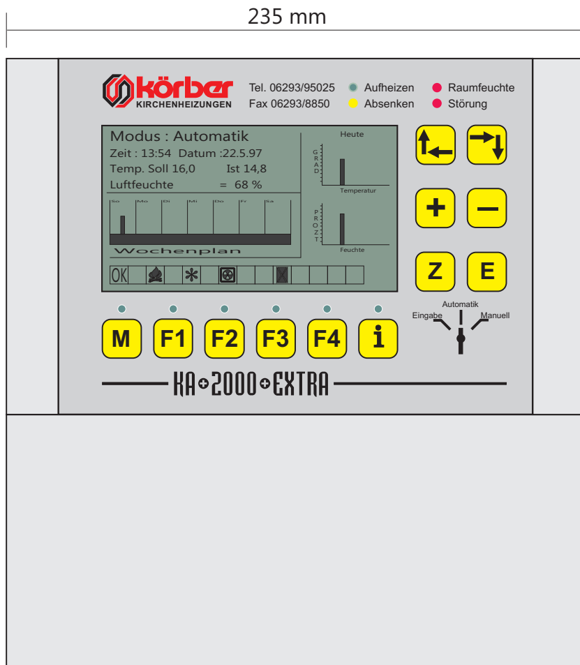
Vorderansicht
